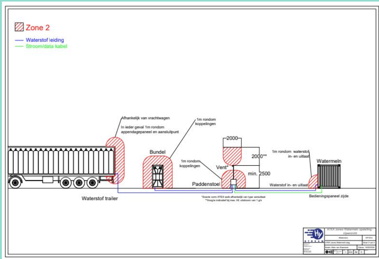
Afbeelding 1: ATEX zonering Watermeln unit gekoppeld aan waterstof bundel of waterstoftank
